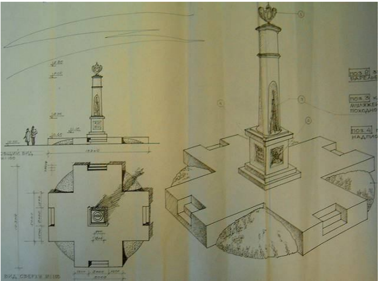
Проект памятника Угличскому полку
