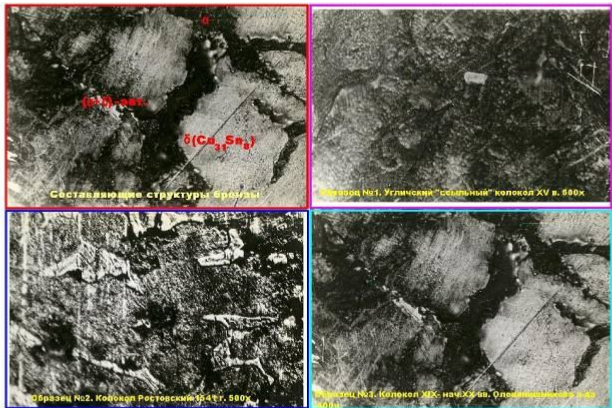
Структура исследованных колокольных сплавов
